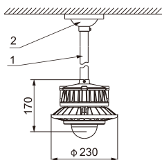
吊杆式安装 (g)
